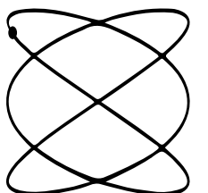
2 Trajektionsmischer J4-Mixer von hs-tumbler mit 4 Mischkammern (links); beispielhafte Mischbahn der Mischkammer (rechts).
