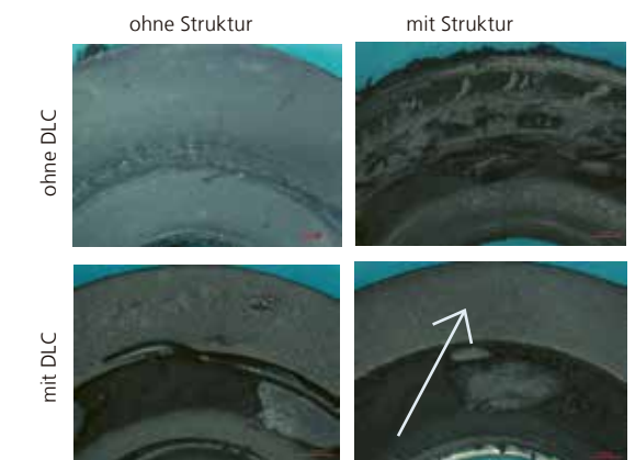
PFAS-freies Elastomer mit DLC-Beschichtung und Laser-Strukturierung (im Vergleich): niedrigster Reibwert (Diagramm oben); kein Verschleiß feststellbar (Aufnahmen unten, blauer Pfeil).
