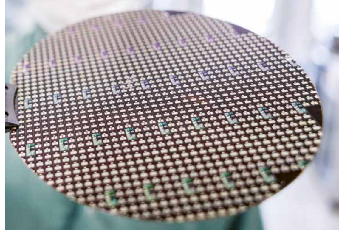
Leistungsbaulemente auf einem Siliziumkarbid-Wafer, hergestellt im institutseigenen Reinraum des Fraunhofer IISB im Rahmen des Projektes »ThinSiCPower«
