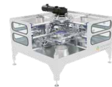
2 Trajektionsmischer J4-Mixer von hs-tumbler mit 4 Mischkammern (links); beispielhafte Mischbahn der Mischkammer (rechts).
