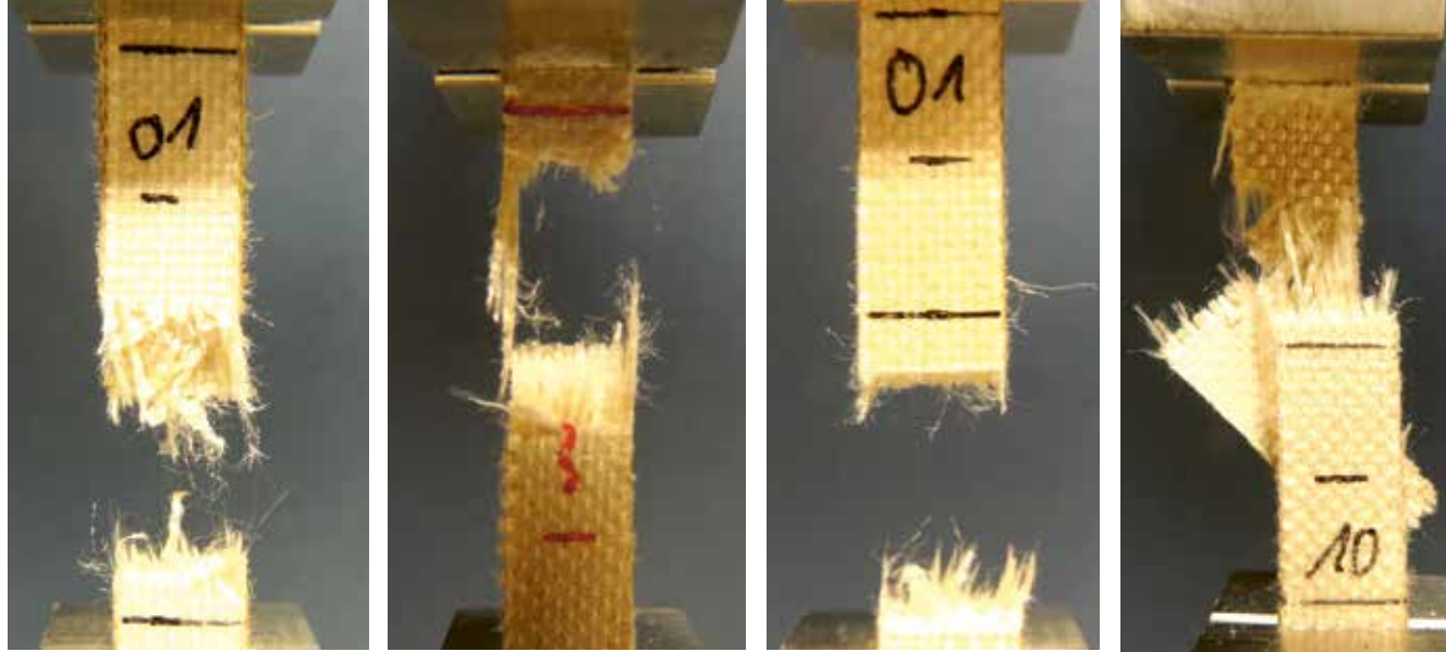
1 Versagensmoden verschiedener naturfaserverstärkter Verbundwerkstoffe
