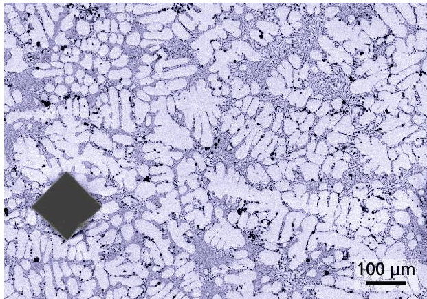
Lichtmikroskopische Aufnahme eines Aluminiumgussgefüges mit dem Eindruck eines Stempels zur Ermittlung der sogenannten Vickershärte (schwarze Raute). (© Fraunhofer-Institut für Werkstoffmechanik IWM)
